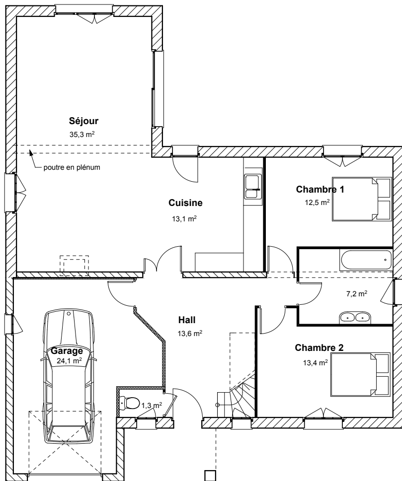
plan RDC
