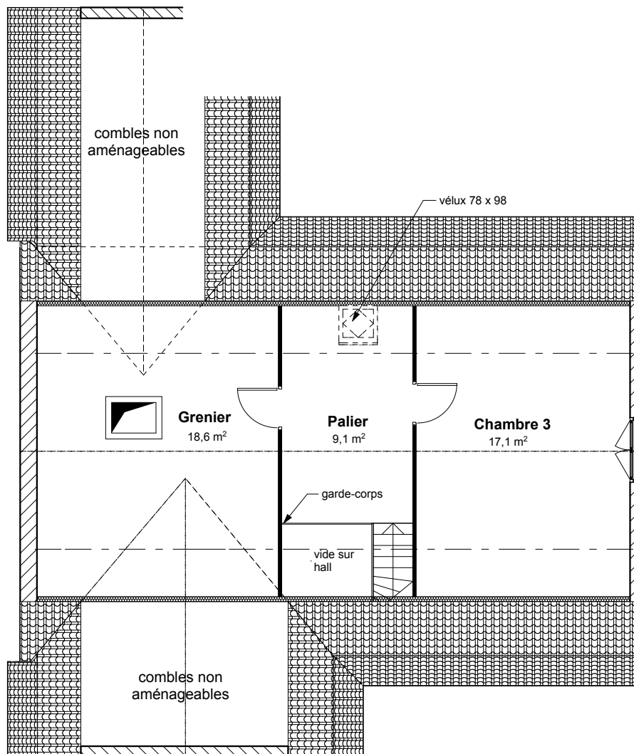
plan étage
