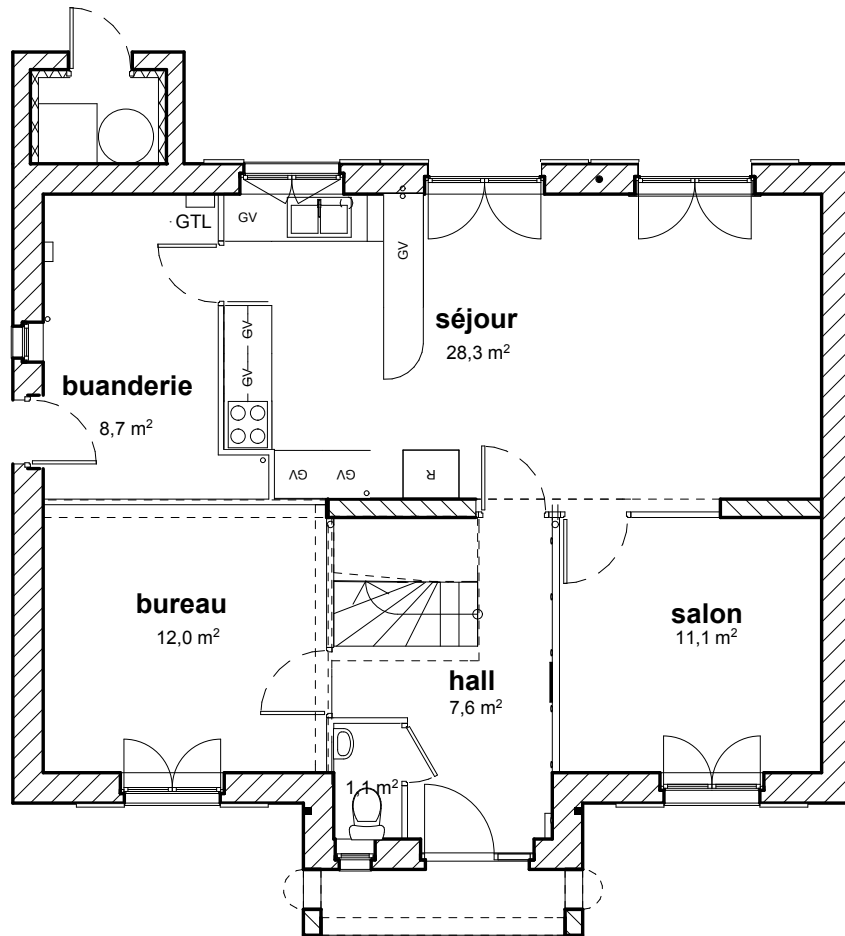
plan RDC
