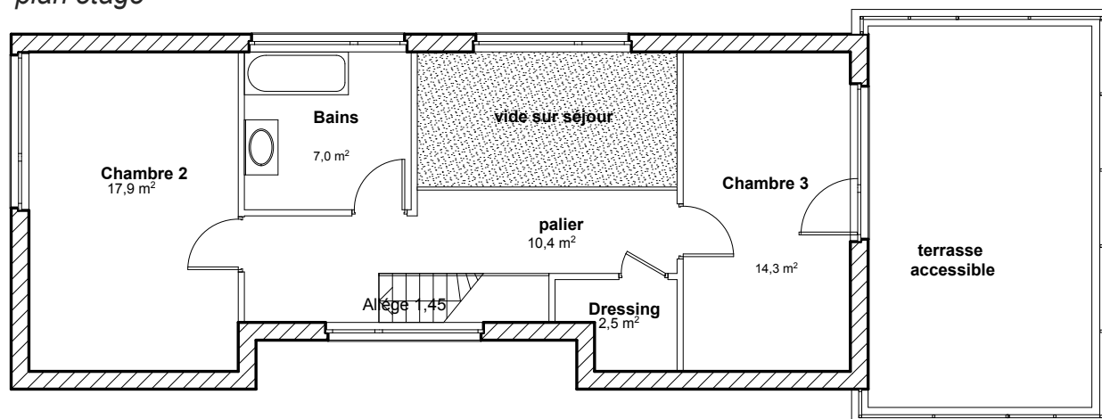
plan étage
